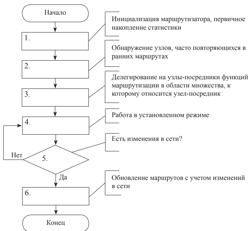
Рис. 2. Схема работы алгоритма самоорганизации сети
