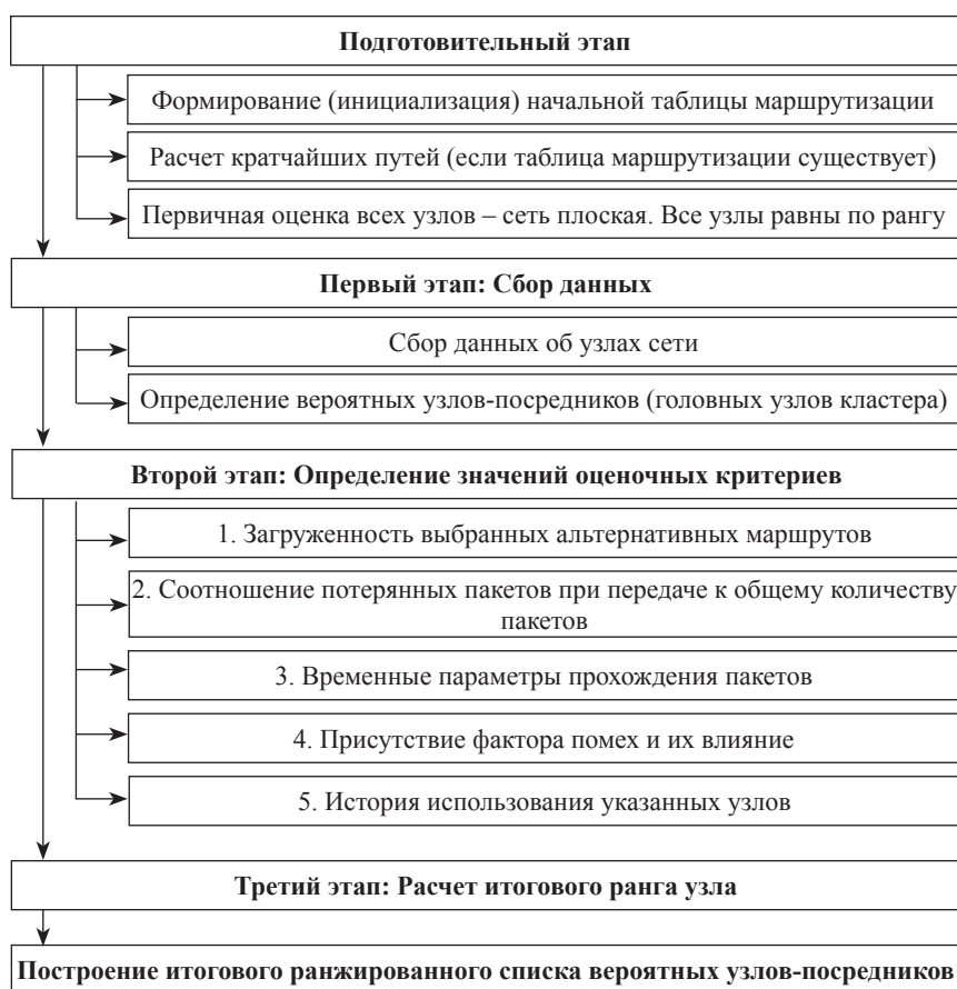
Рис. 1. Структурная схема процесса ранжирования узлов
